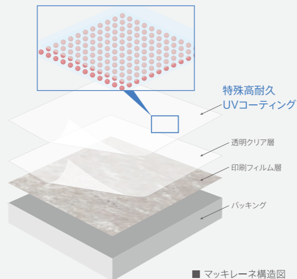
■ マッキレーネ構造図
